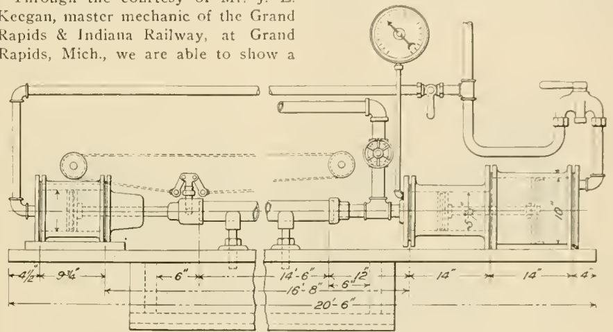
FLUE TESTING APPARATUS.
